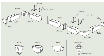
標準組立図
