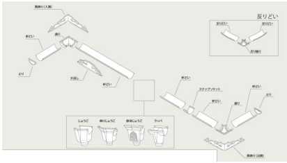
標準組立図
