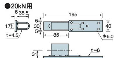
ビスどめホールダウンU-20KN
