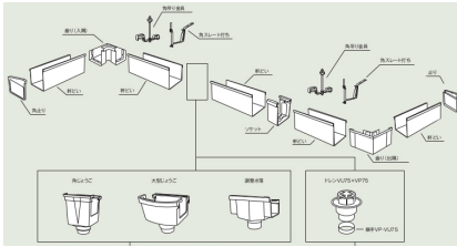
標準組立図
