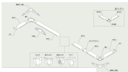
標準組立図
